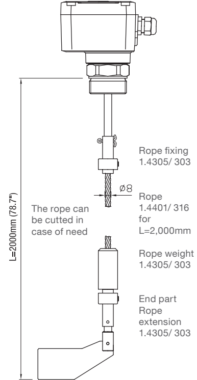
pos.39 Kit „rope extension"
