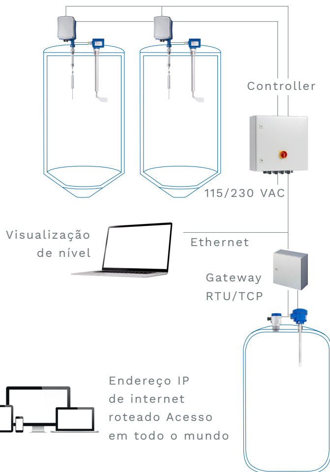
Esquema exemplar de planejamento de projeto NT 3500 / 4500
